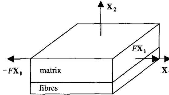
Figure 3.1. Longitudinal tension
