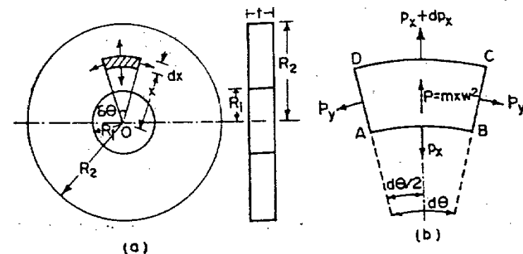
Fig. 18.2. Rotating disc.
