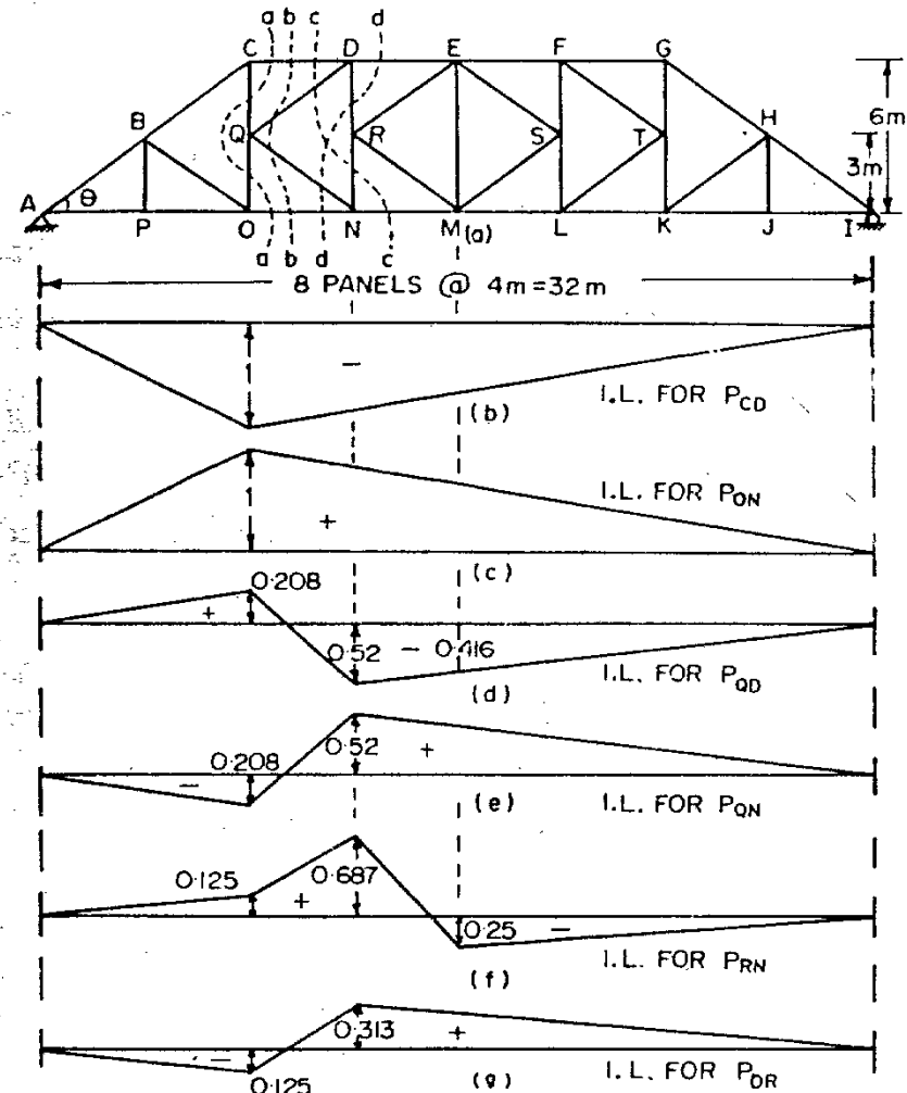
Fig. 4.4 K-Truss
