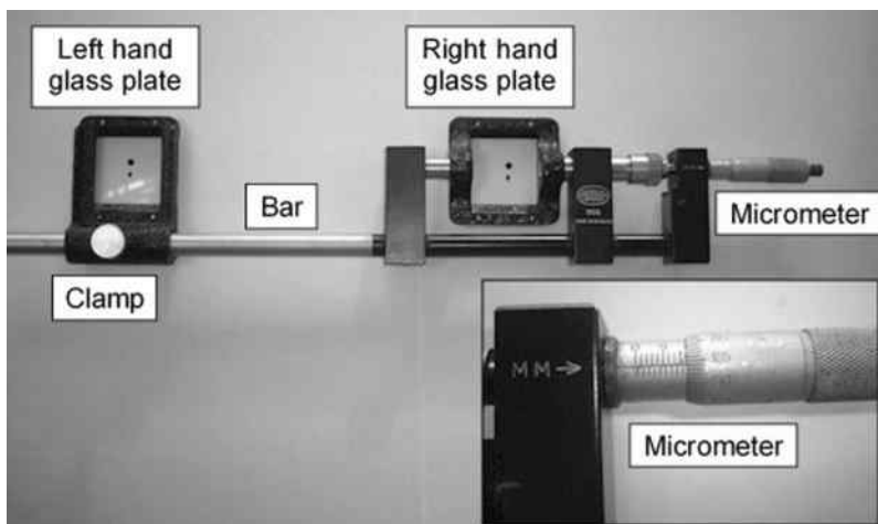
Fig. 14.25 Parallax bar
