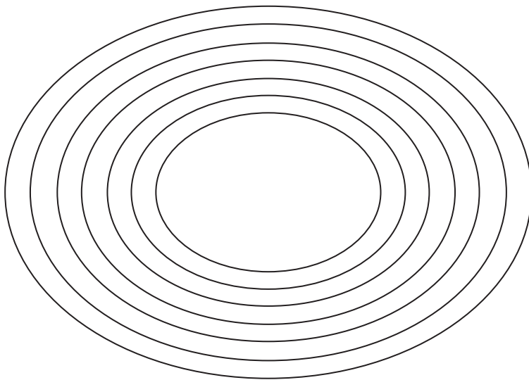
Fig. 8.3 Equipotential surfaces
