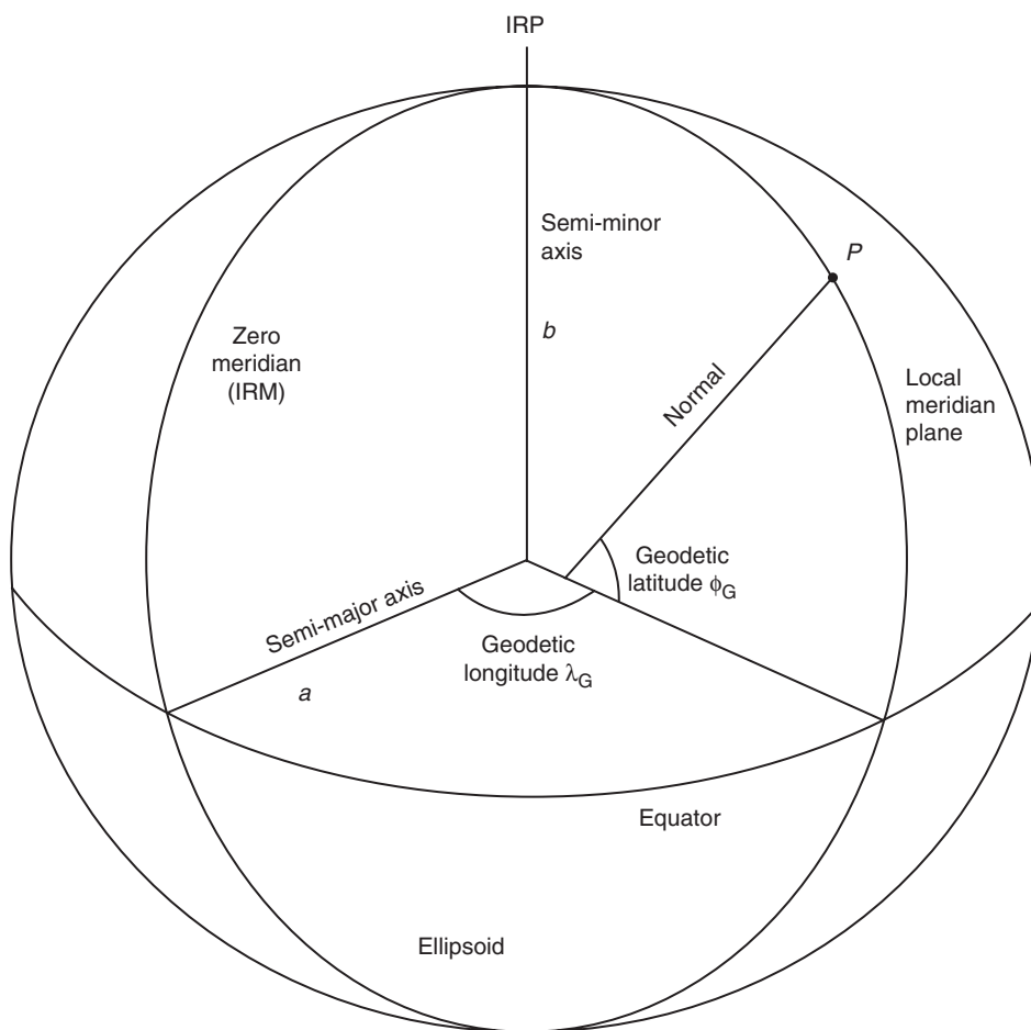
Fig. 8.7 Geodetic coordinates
