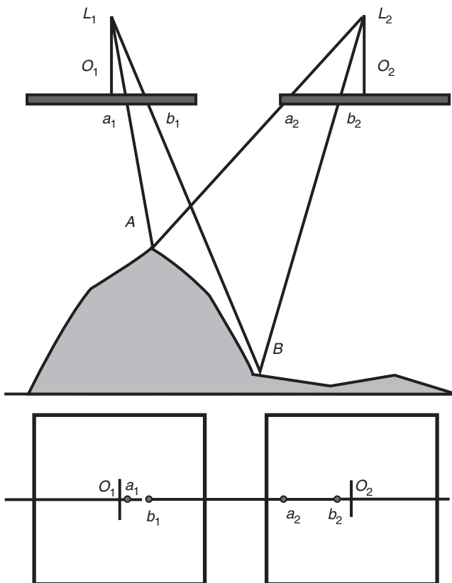
Fig. 14.3 Parallax
