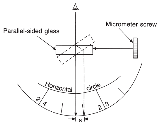
Fig. 5.5 Micrometer
