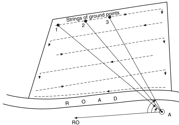
Fig. 3.48 Plotting
