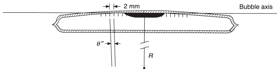
Fig. 3.12 Tubular bubble
