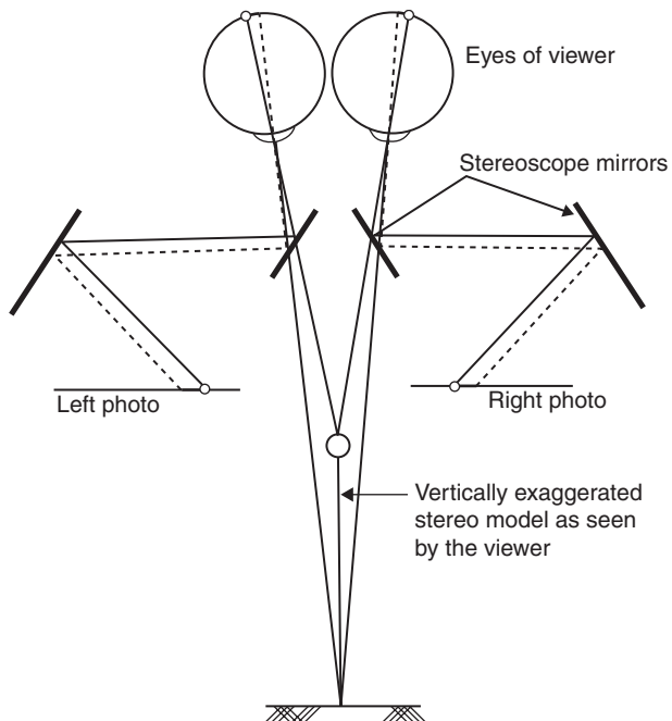
Fig. 14.23 Stereoscope
