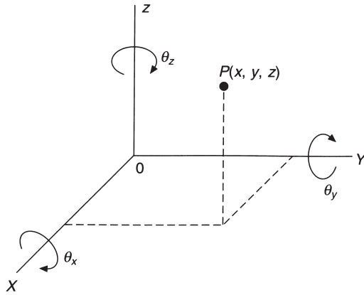
Fig. 8.14 Transformation parameters
