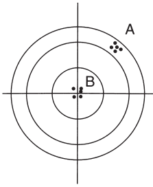
Fig. 2.1 Scatter
